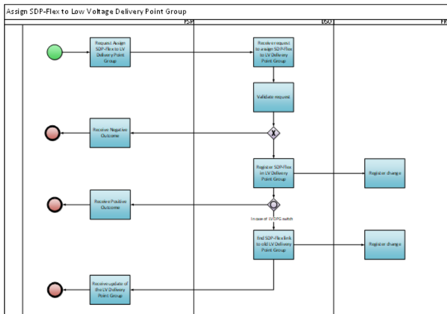
Figure 25 - Attribution d'un SDP Flex à un DPG
