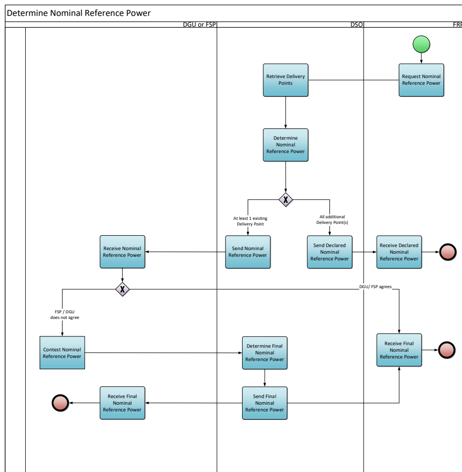
Figure 16 - Calcul de la Puissance nominale de référence
