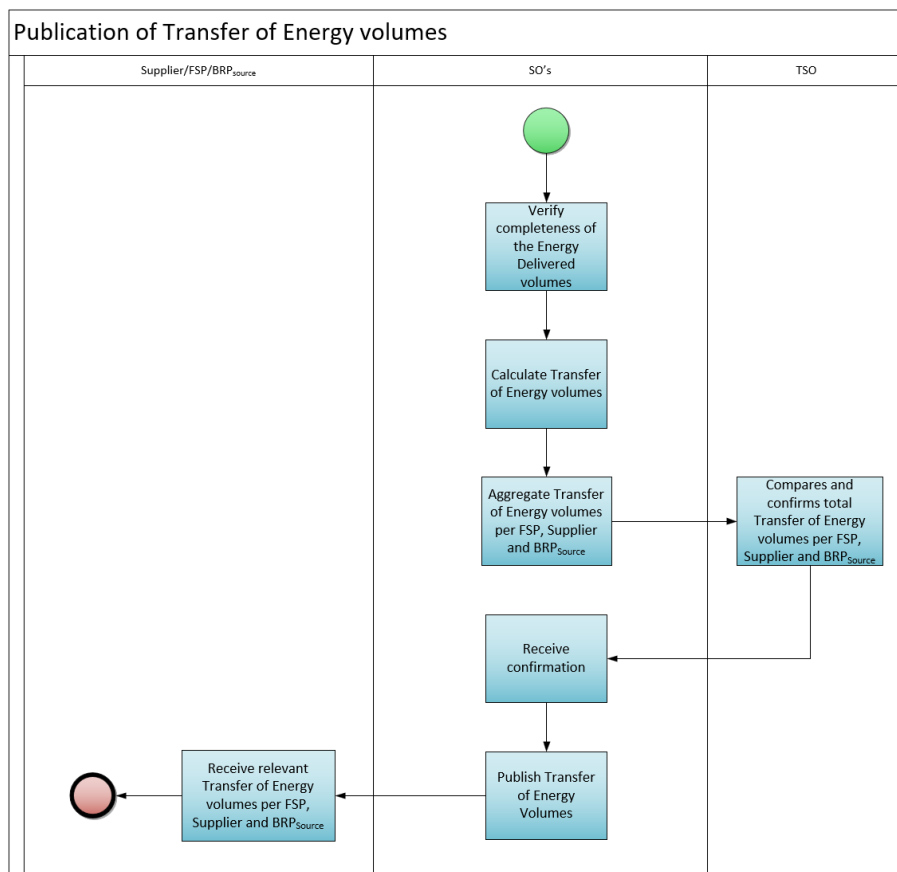
Figure 21 - Publication des volumes d'énergie transférée
