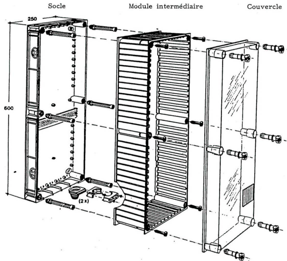
Figure 5.1 - Coffret de comptage standard pour une installation \leq 63A dans un immeuble unifamilial
